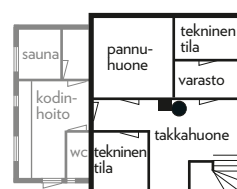
POHJAKERROS
